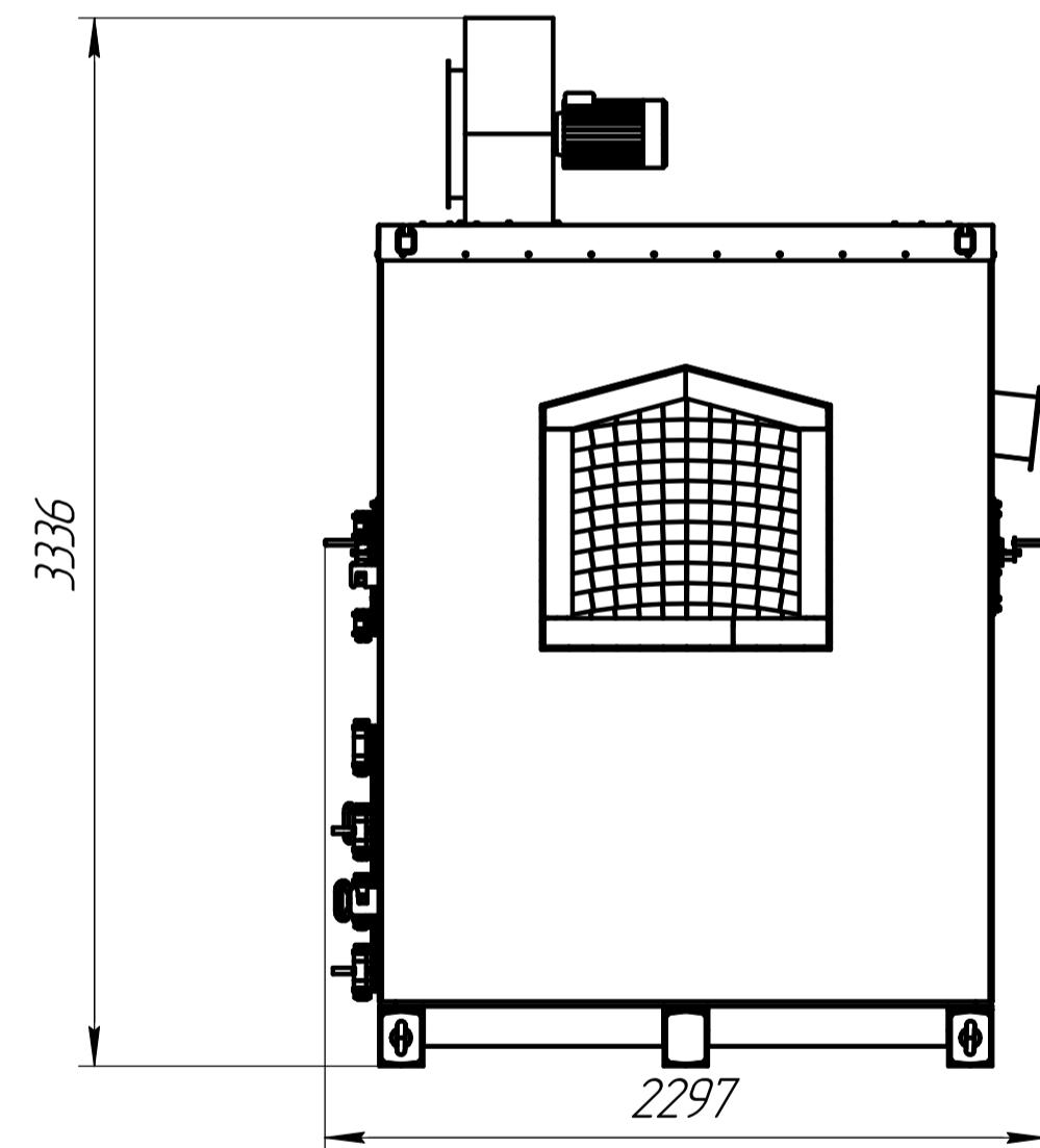
"Дракон Мега" – 4 МВт Масса – 13800 кг
