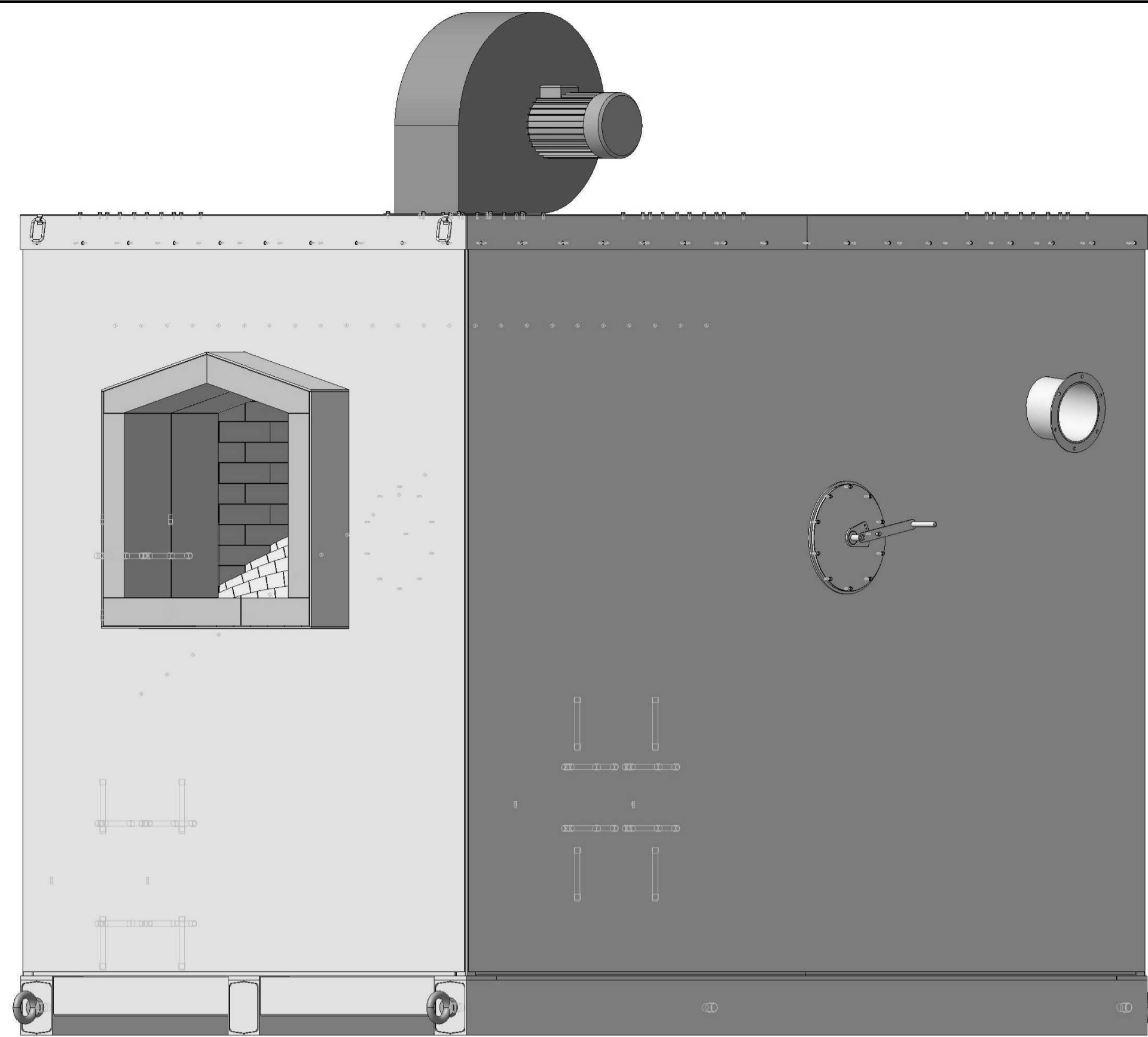
"Дракон Мега" – 4 МВт Масса – 13800 кг
